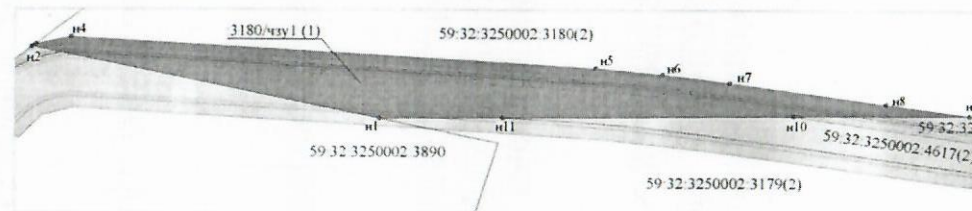
Схема части земельного участка :3180/чзу1(1) М 1:1000
